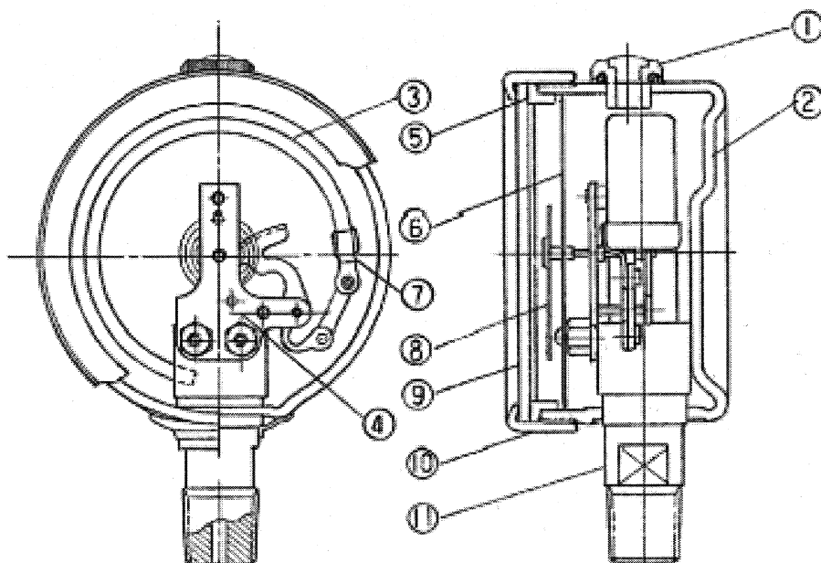
図 6-1 構造図
